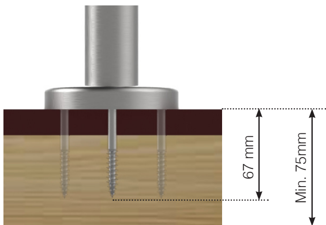
SKRUE FOR INNFESTING I TRE
